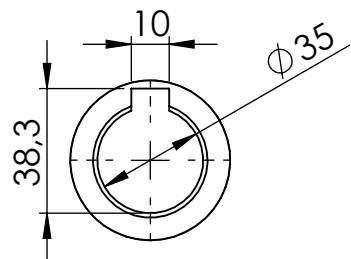
DETAY A
